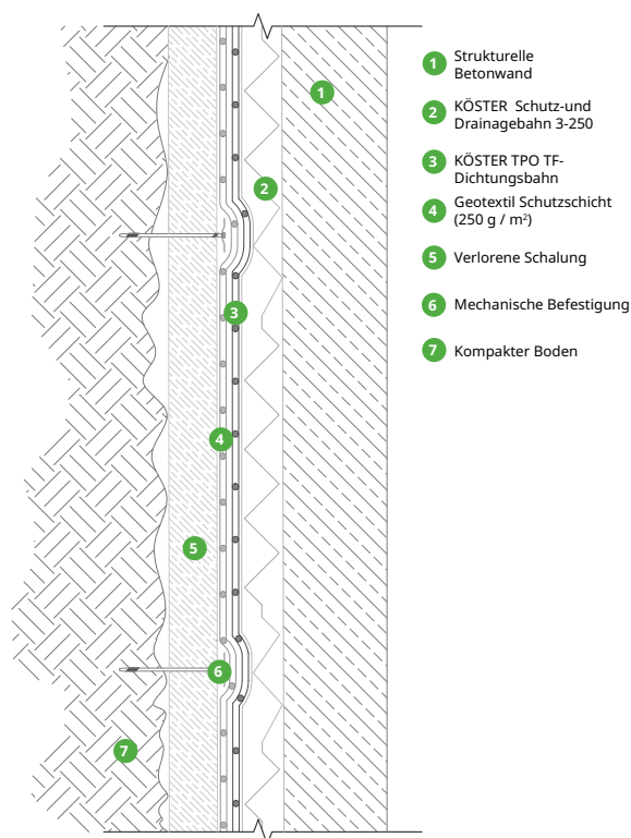
Abdichtung verlorener Schalung mit KÖSTER TPO TF-Dichtungsbahnen
